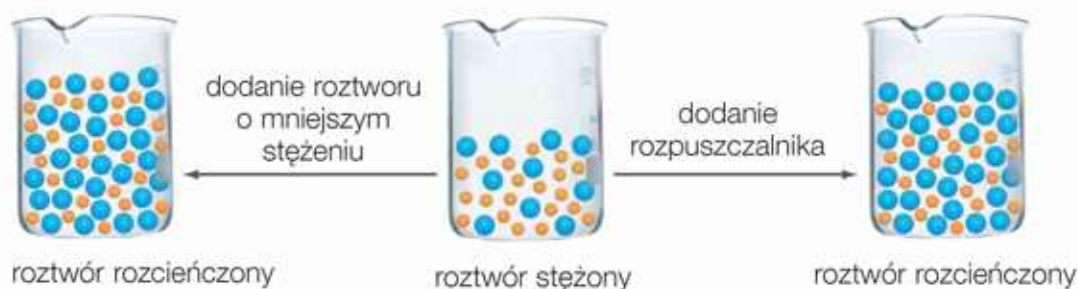
Rys. 37. Sposoby zmniejszania stężenia roztworu.
