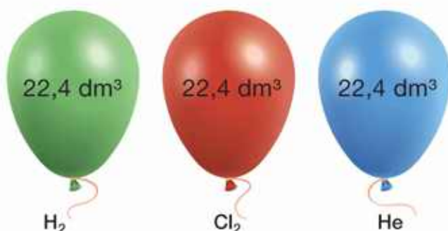
Rys. 21. W warunkach normalnych objętość molowa różnych gazów jest taka sama i wynosi 22,4 \text{ dm}^3 .
