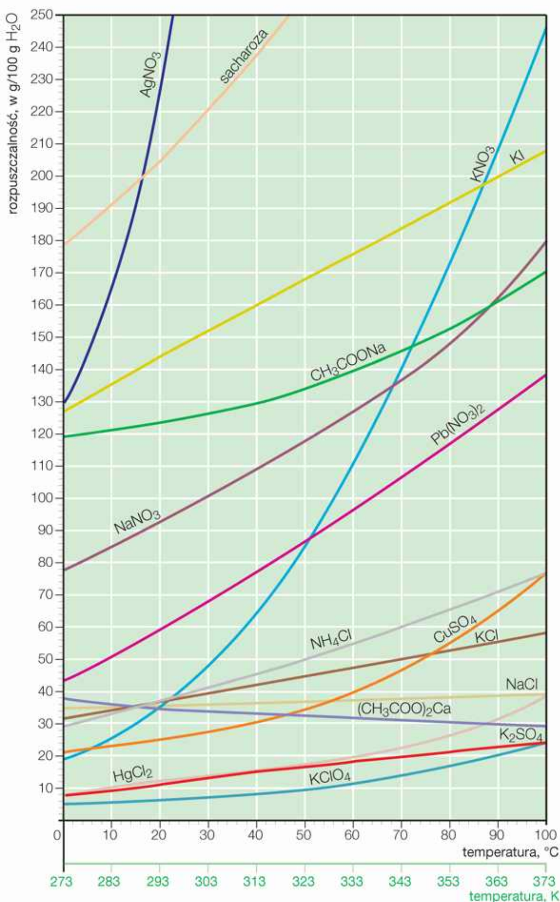
Rys. 34. Krzywe rozpuszczalności – zależność rozpuszczalności substancji stałych w wodzie od temperatury: AgNO 3 – azotan(V) srebra(I); KI – jodek potasu; NaNO 3 – azotan(V) sodu; KNO 3 – azotan(V) potasu; Pb(NO 3 ) 2 – azotan(V) ołowiu(II); NH 4 Cl – chlorek amonu; CuSO 4 – siarczan(VI) miedzi(II); K 2 SO 4 – siarczan(VI) potasu; KCl – chlorek potasu; NaCl – chlorek sodu; (CH 3 COO) 2 Ca – etanian (octan) wapnia; CH 3 COONa – etanian (octan) sodu; HgCl 2 – chlorek rtęci(II); KClO 4 – chloran(VII) potasu; sacharoza – C 12 H 22 O 11 .
