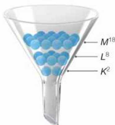
Rys. 6. Na najniższym poziomie mieszczą się 2 elektrony, co odpowiada pierwszej powłoce elektronowej K . Następne warstwy odpowiadają kolejnym powłokom elektronowym: L i M , w których może znajdować się odpowiednio 8 i 18 elektronów.
