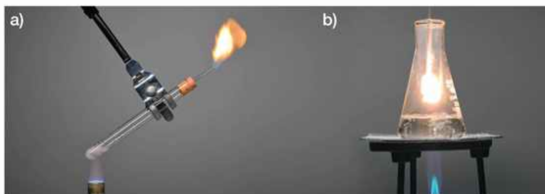
Fot. 6. Ogrzewanie substancji znajdujących się w: a) probówce, b) kolbie stożkowej.
