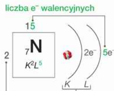
Rys. 4. Schemat rozmieszczenia powłok elektronowych wokół jądra atomowego.
