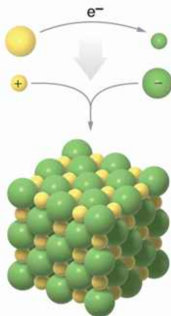
Rys. 12. Model powstawania kryształu jonowego chlorku sodu.
