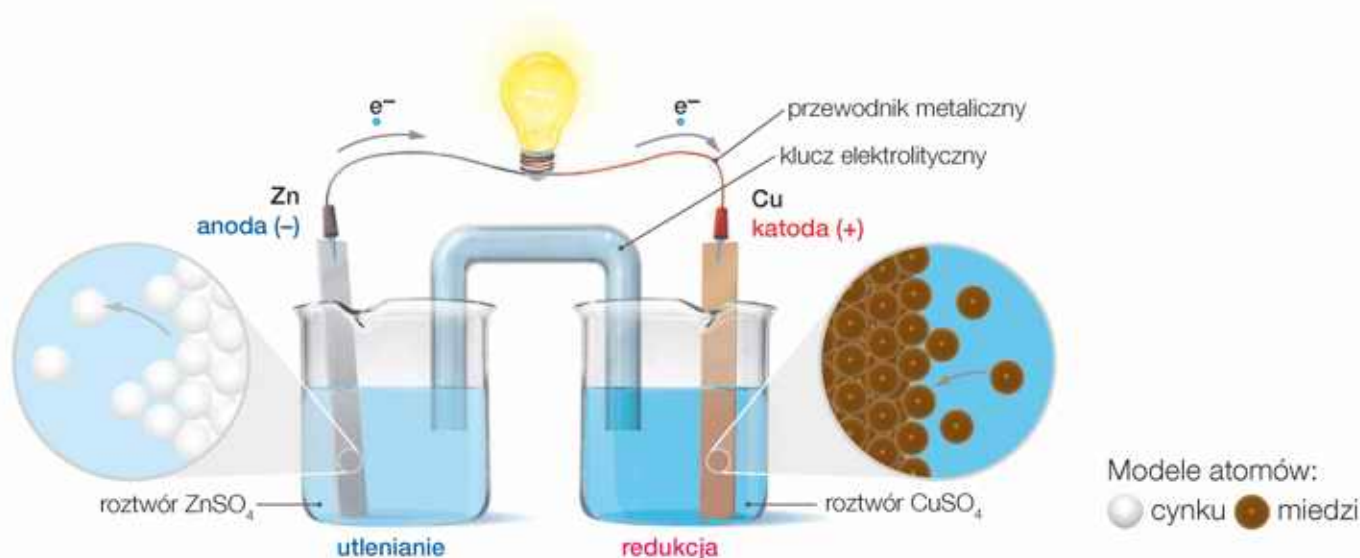
Rys. 27. Reakcje zachodzące w ogniwie Daniella.
