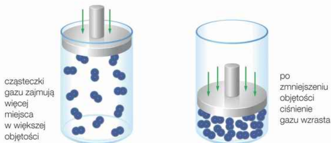
Rys. 20. Im mniejszą przestrzeń (objętość) zajmują cząsteczki gazu, tym wyższe ciśnienie panuje w zbiorniku.
