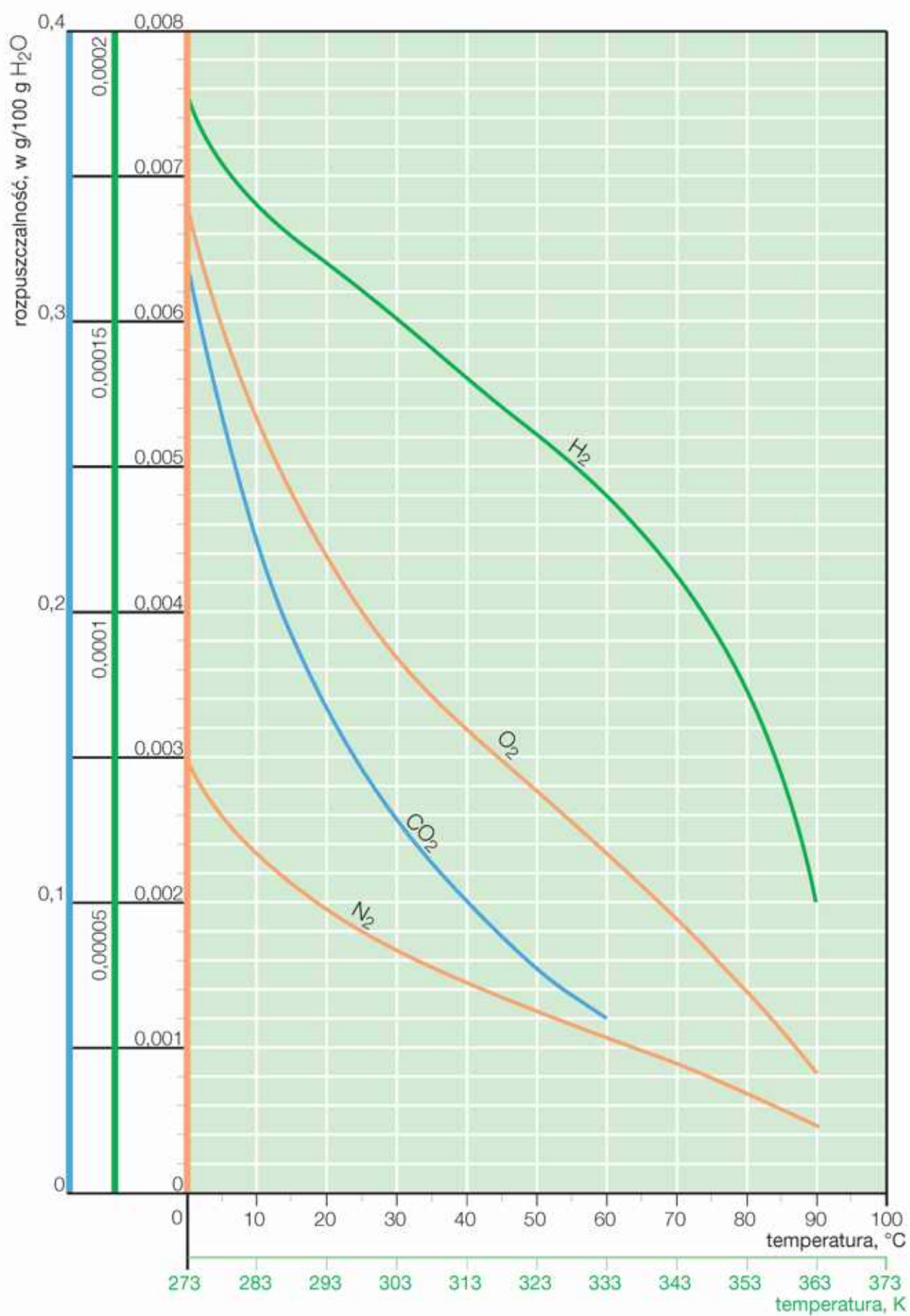
Rys. 35. Krzywe rozpuszczalności – zależność rozpuszczalności gazów w wodzie od temperatury.
