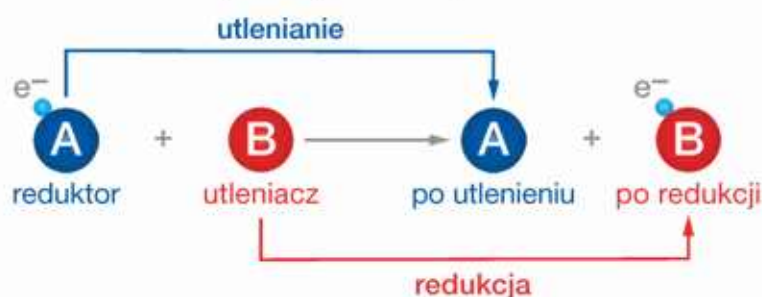
Rys. 23. Model reakcji utleniania-redukcji.
