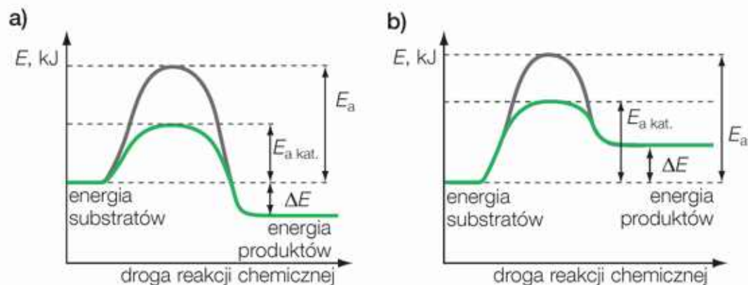
Rys. 49. Wykres zmian energii dla reakcji: a) egzotermicznej, b) endotermicznej, przebiegających bez udziału katalizatora i z jego udziałem, gdzie: E_a – energia aktywacji reakcji chemicznej bez udziału katalizatora, E_{a \text{ kat.}} – energia aktywacji reakcji chemicznej z udziałem katalizatora, \Delta E – energia wydzielana lub pobierana przez układ. Efekt energetyczny reakcji chemicznej: — bez udziału katalizatora, — z udziałem katalizatora.
