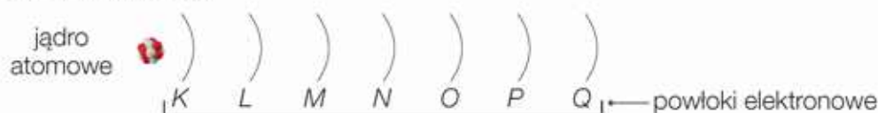
Rys. 4. Schemat rozmieszczenia powłok elektronowych wokół jądra atomowego.
