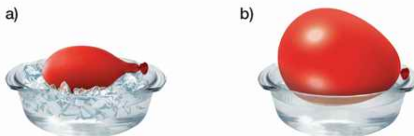
Rys. 19. Cząsteczki gazu w balonie umieszczonym w naczyniu z lodem (a) poruszają się wolniej i zajmują mniejszą przestrzeń niż cząsteczki tego samego gazu w gorącej wodzie (b).
