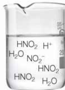
słaby elektrolit
