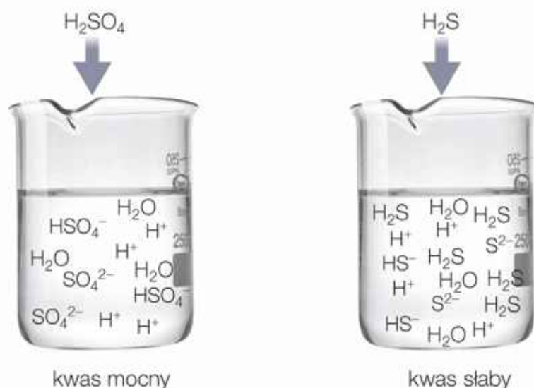
Rys. 18. W roztworze kwasu mocnego występują wyłącznie jony, w roztworze kwasu słabego – zarówno jony, jak i cząsteczki.
