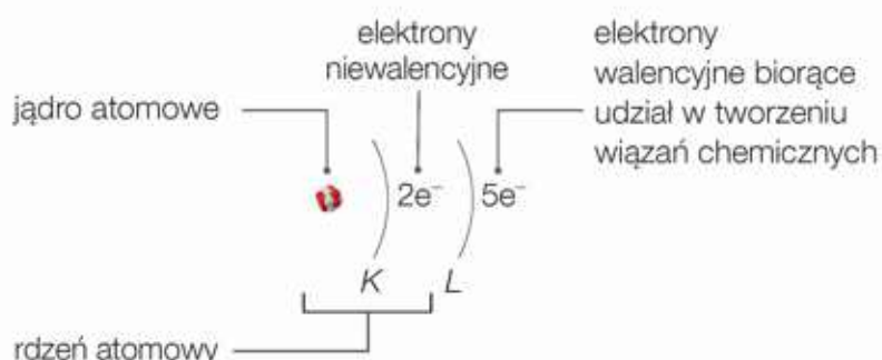
Rys. 5. Uproszczony model atomu azotu.
