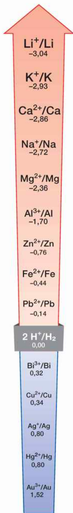
Rys. 26. Szereg elektrochemiczny (napięciowy) metali.
