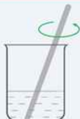
mieszanie
