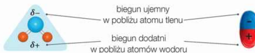
Rys. 10. Cząsteczka wody jest dipolem – ma budowę polarną.
