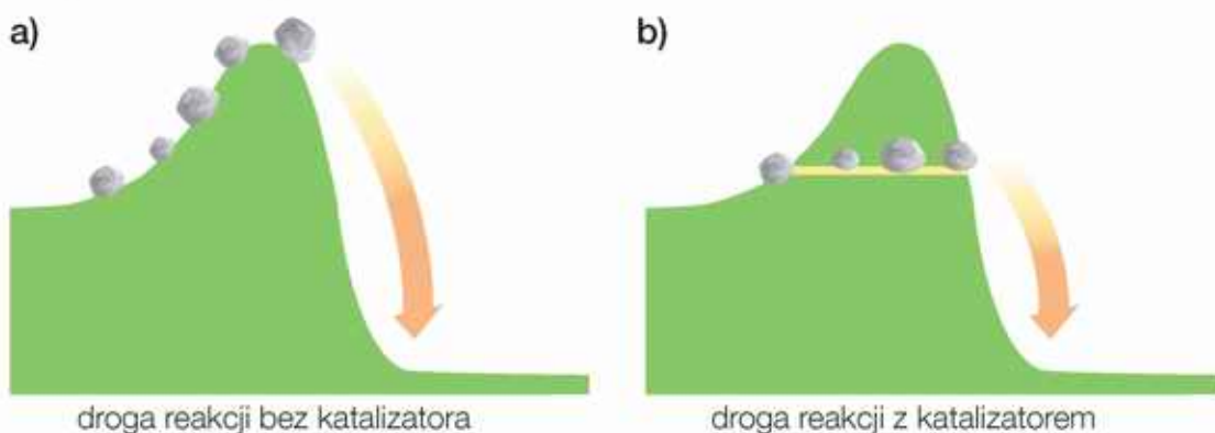
Rys. 48. Reakcja chemiczna bez udziału katalizatora wymaga dostarczenia większej ilości energii (a) niż reakcja chemiczna z udziałem katalizatora (b).
