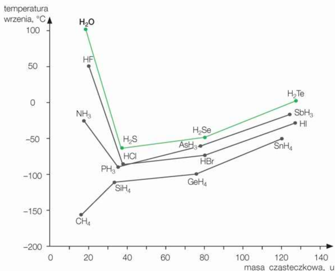
Rys. 14. Zależność temperatur wrzenia substancji od ich masy cząsteczkowej.
