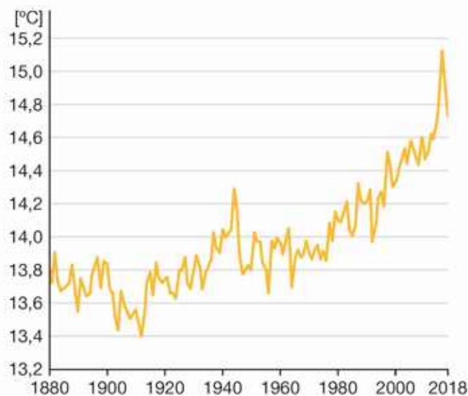
Średnia roczna temperatura powietrza na Ziemi w latach 1880–2018.
