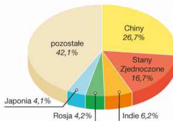
Udział największych producentów w światowej produkcji energii elektrycznej w 2018 r.
