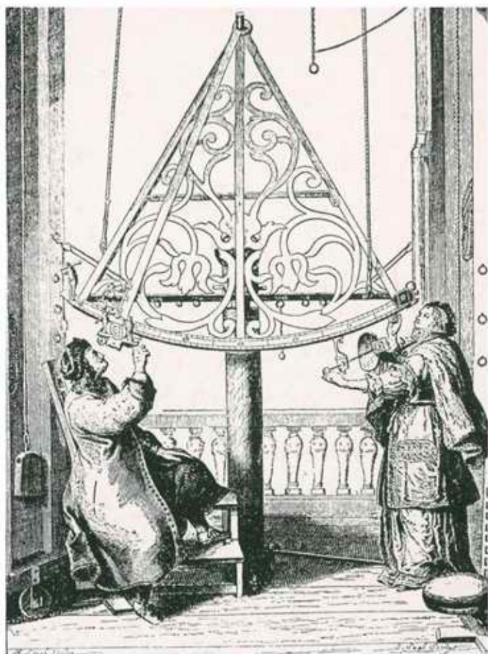
Jan Heweliusz i jego żona Elżbieta Koopman przy pracy – rycina przedstawia małżeństwo gdańskich uczonych obserwujące niebo. Jednym z odkryć Heweliusza jest gwiazdozbiór Tarcza Sobieskiego, któremu nazwę nadał dla uczczenia wielkiego zwycięstwa pod Wiedniem.
