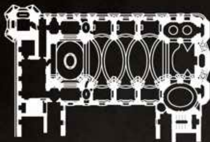
Rzut poziomy kościoła św. Mikołaja w Pradze
